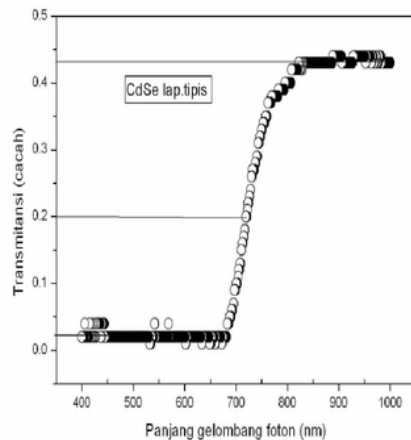
Gambar 5. Transmittansi CdSe pada panj. glb. antara 400 nm sampai 1000 nm.
