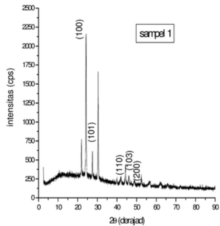
Gambar 2. Difraktogram lapisan tipis CdSe
