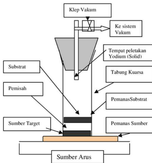
Gambar 1. Skema teknik CSVT.
